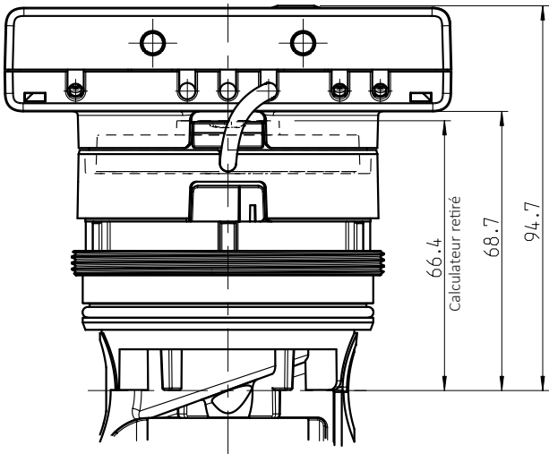
SensoStar 3 jets multiples / détachable
