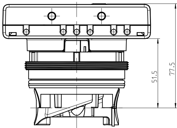
SensoStar 3 flujo múltiple / compacto
