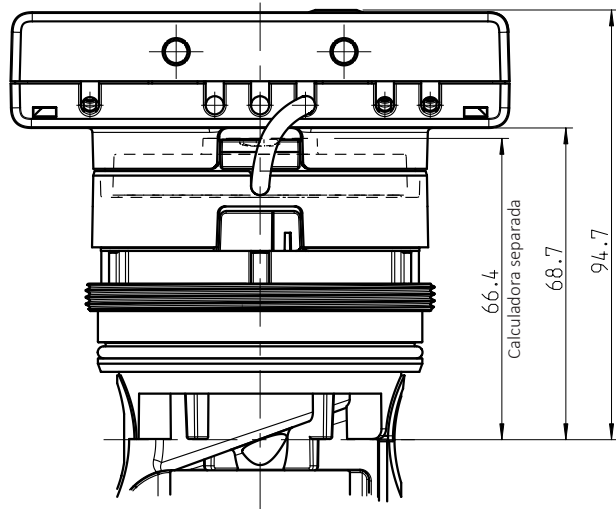
SensoStar 3 flujo múltiple / separable
